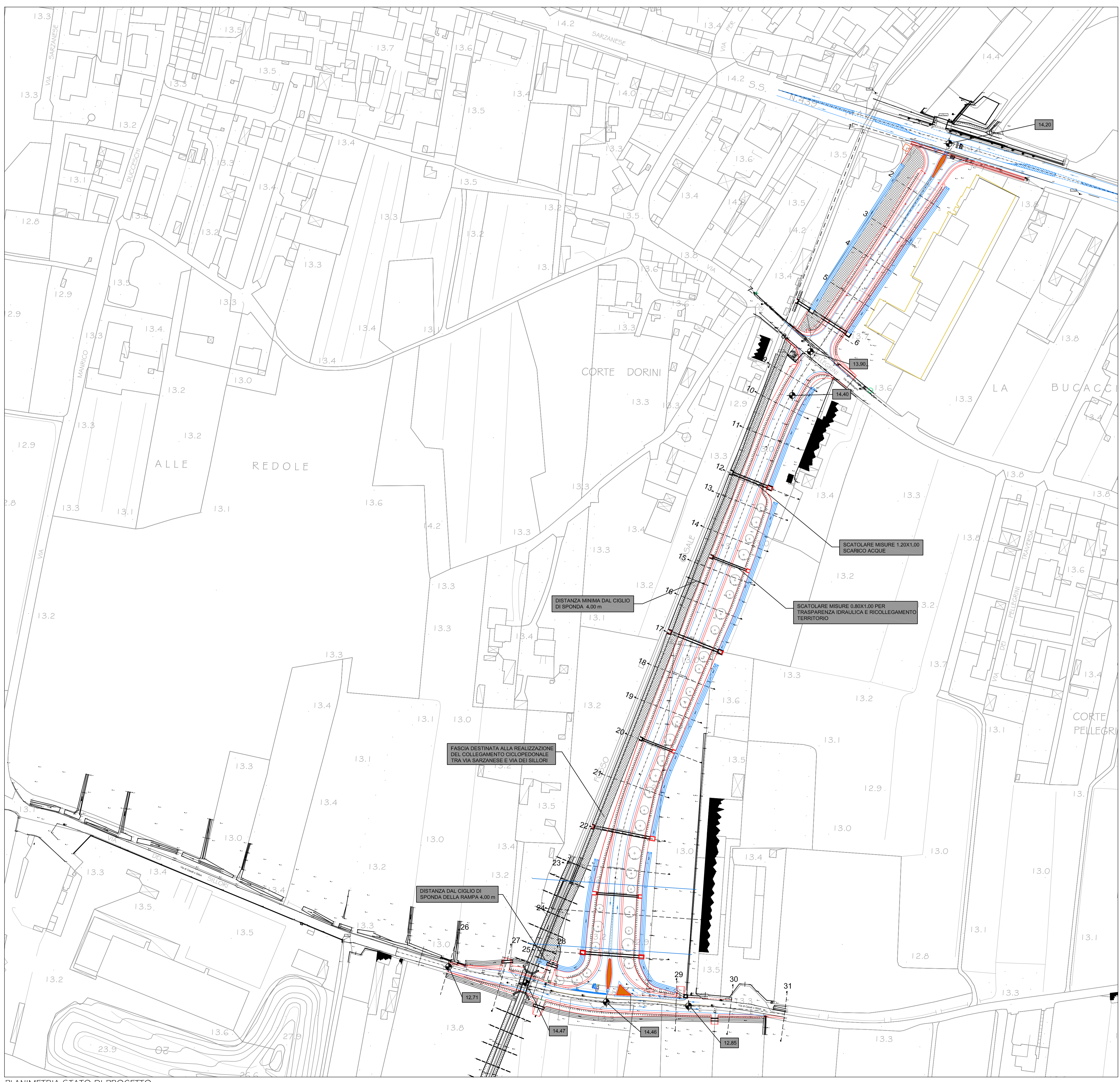
PLANIMETRIA STATO DI PROGETTO
