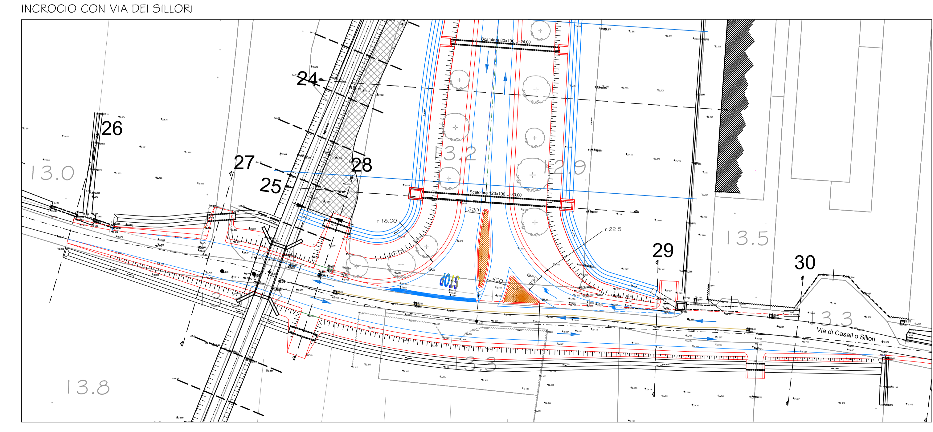
INCROCIO CON VIA SARZANESE
