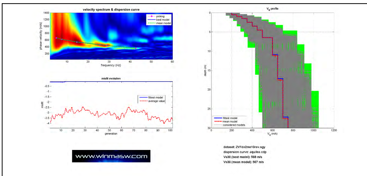
Fig.2: Grafico Misfit - Profilo verticale delle Onde S
