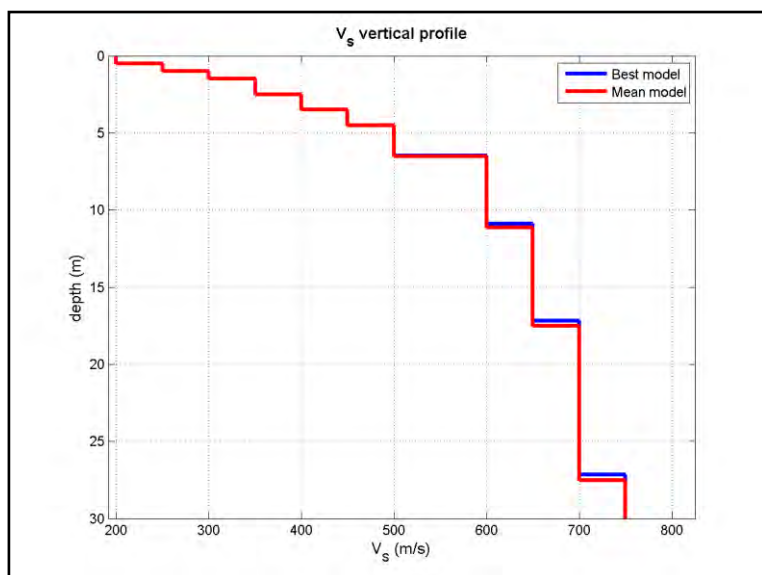
Fig.3: Profilo verticale Vs (Modello medio/Modello migliore)
