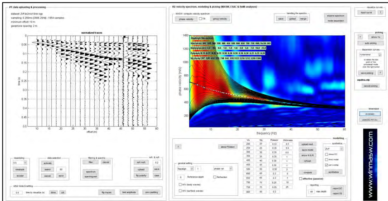
Fig.1: Sismogramma (Shot1 ZVfDx2mo10rev) e spettro delle velocità con "picking"
